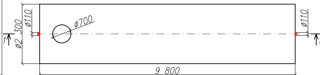
Вид сверху
