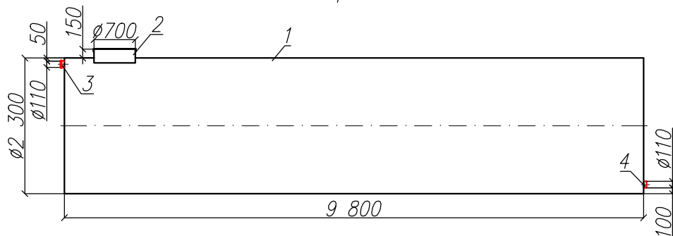
Разрез 1-1
